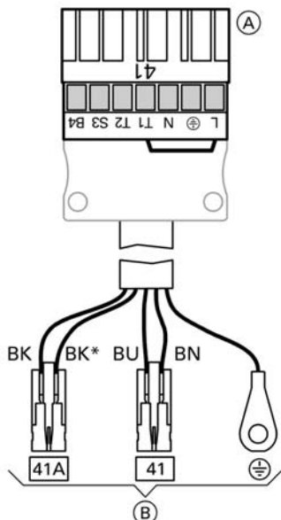
5-жильный кабель горелки
