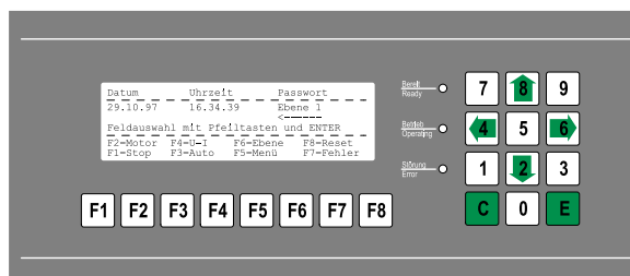
Рис. 16 Меню для ввода пароля: Выбор значения (текущий уровень) имеет двойное подчеркивание (после подтверждения выбора поля с одинарным подчеркиванием клавишей E), после ввода подтвердить цифровую последовательность пароля (для уровня 3) клавишей E
