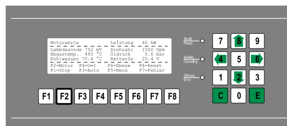
Рис. 24 Отображение параметров двигателя с помощью функциональной клавиши F2; возврат к основному экрану клавишей C (цифровое поле)
