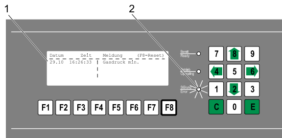
Рис. 26 Квитирование ошибок функциональной клавишей F8
