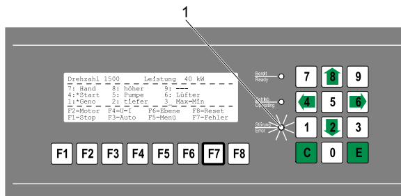
Рис. 25 Отображение списка ошибок с помощью функциональной клавиши F7
