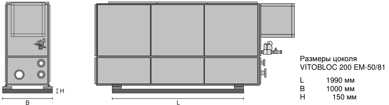
Рис. 7 Размер цоколя
